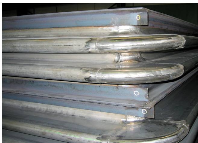
Detail hoekstukken Balgelement: 1.4571 Flenzen: S235JR
