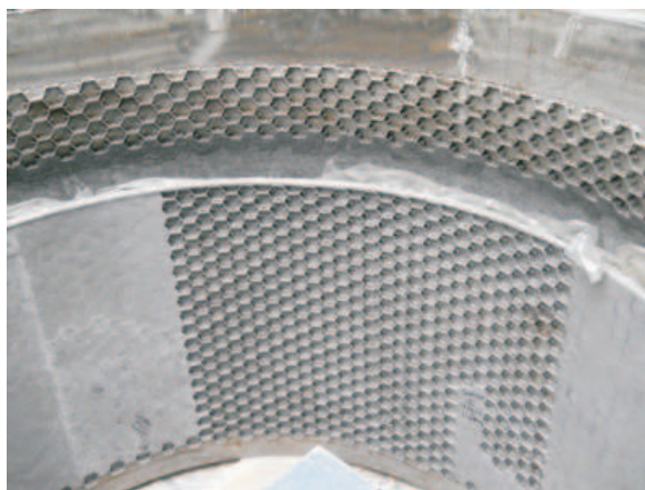
Hexmesh en refractory liner
